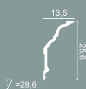
C340 200 x 25,6 x 13,5 cm Purotouch ®
