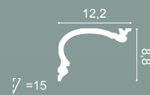
C341 | C341F HERITAGE 200 x 8,8 x 12,2 cm Purotouch ®
